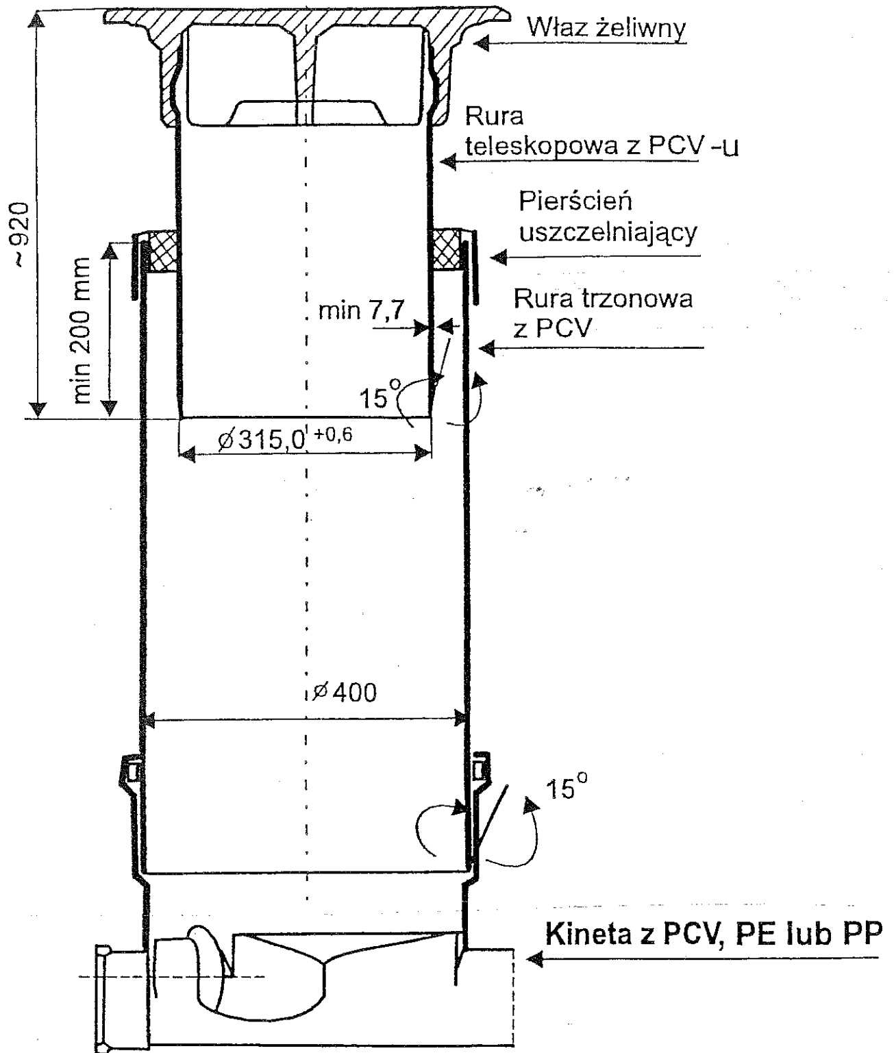
Przykład studzienki kanalizacyjnej z tworzywa sztucznego
